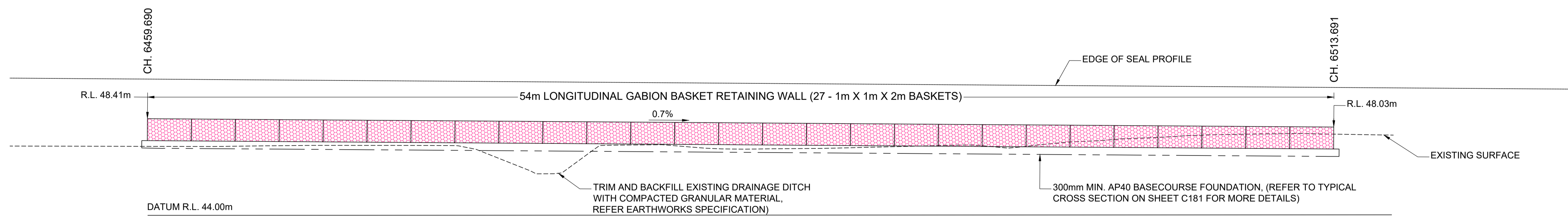
LONGITUDINAL SECTION - L1 Scale: 1:100
